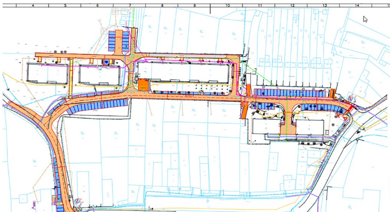
Obrázek č. 2 – Návrh etapizace opravy komunikace u bytovek
