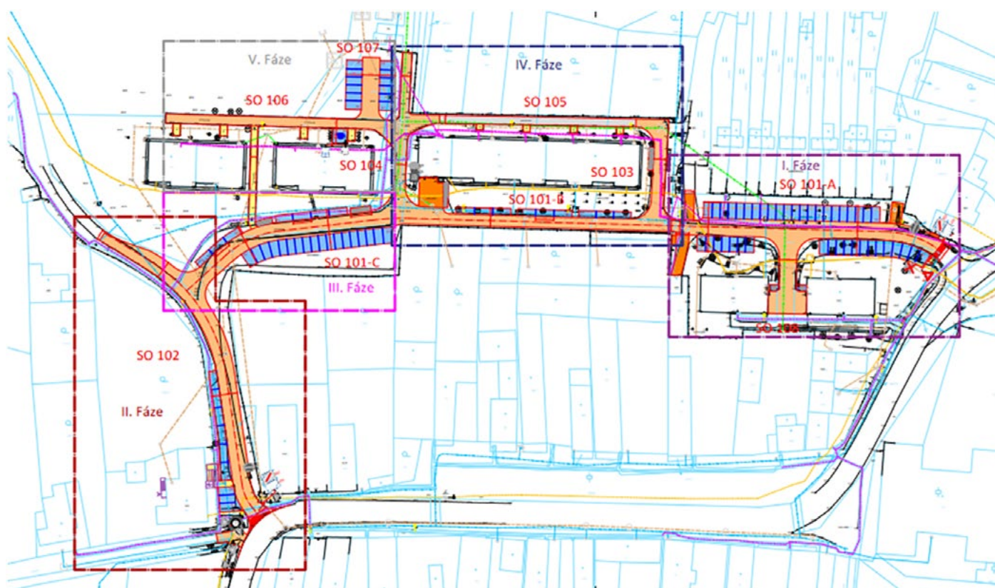
Obrázek č. 2 – Návrh etapizace opravy komunikace u bytovek
